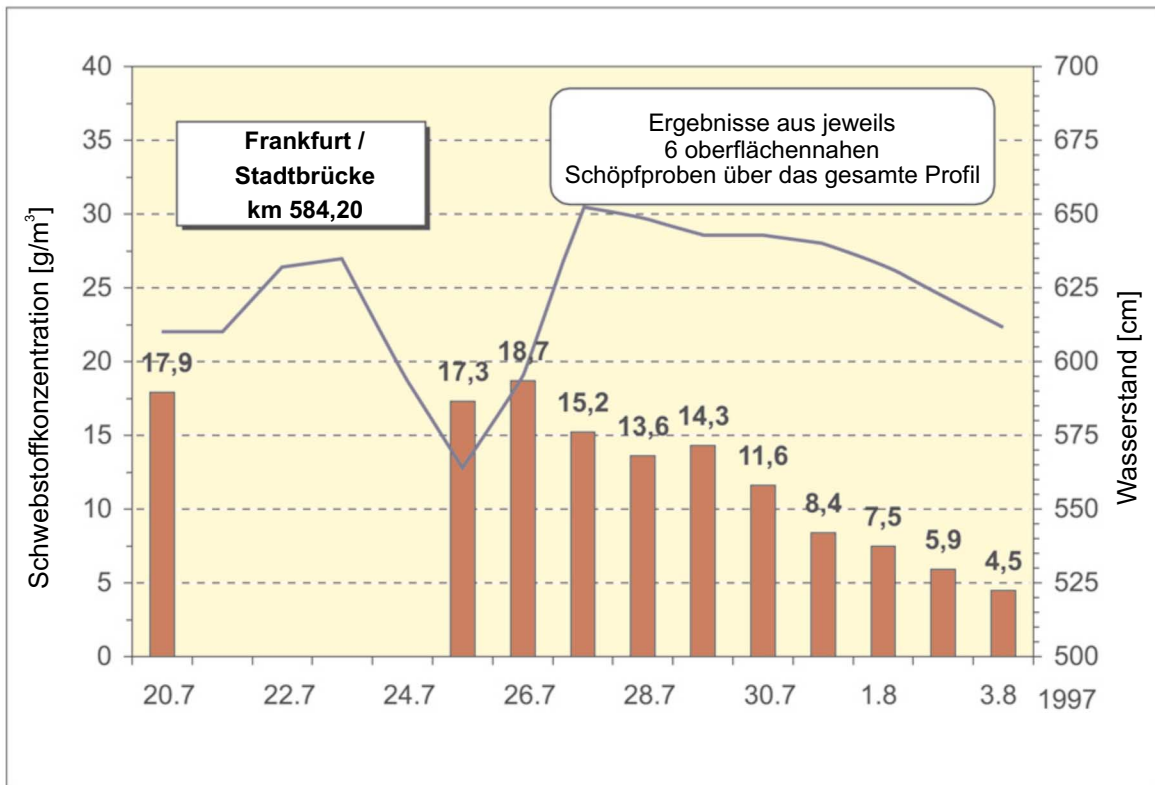
Abb. 8.6a Verlauf der Schwebstoffkonzentration der Oder bei Frankfurt während des Hochwassers
