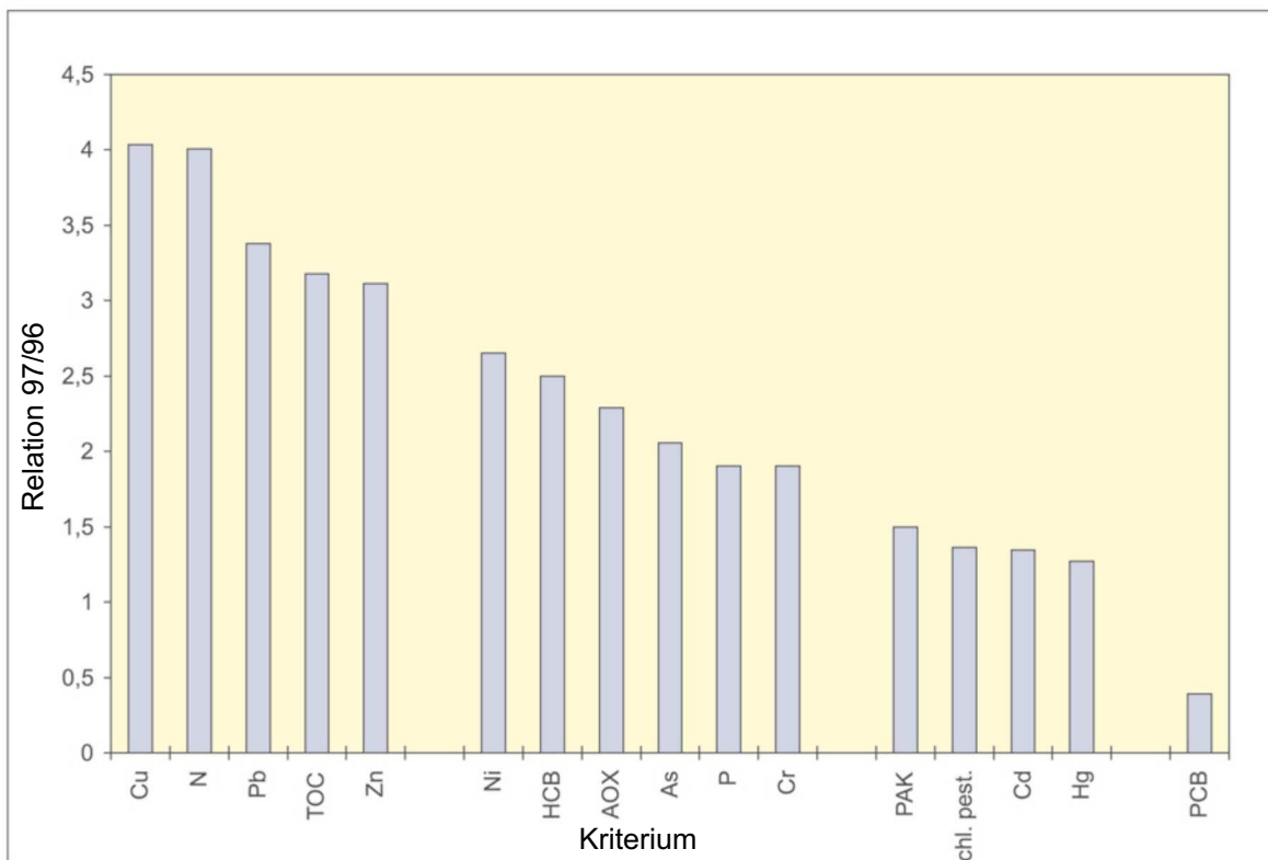
Abb. 9.5 Vergleiche der mittleren Monatsfracht 1996 und der Hochwasserfracht 1997 in Schwedt
