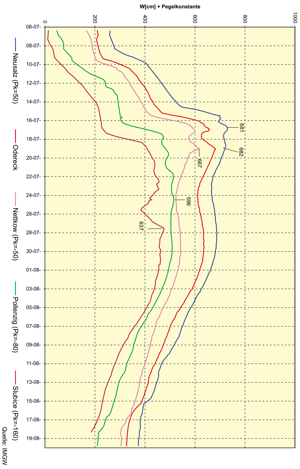
Abb. 4.7 Wasserstandsganglinien für den Oberabschnitt von Neusalz bis Slubice
