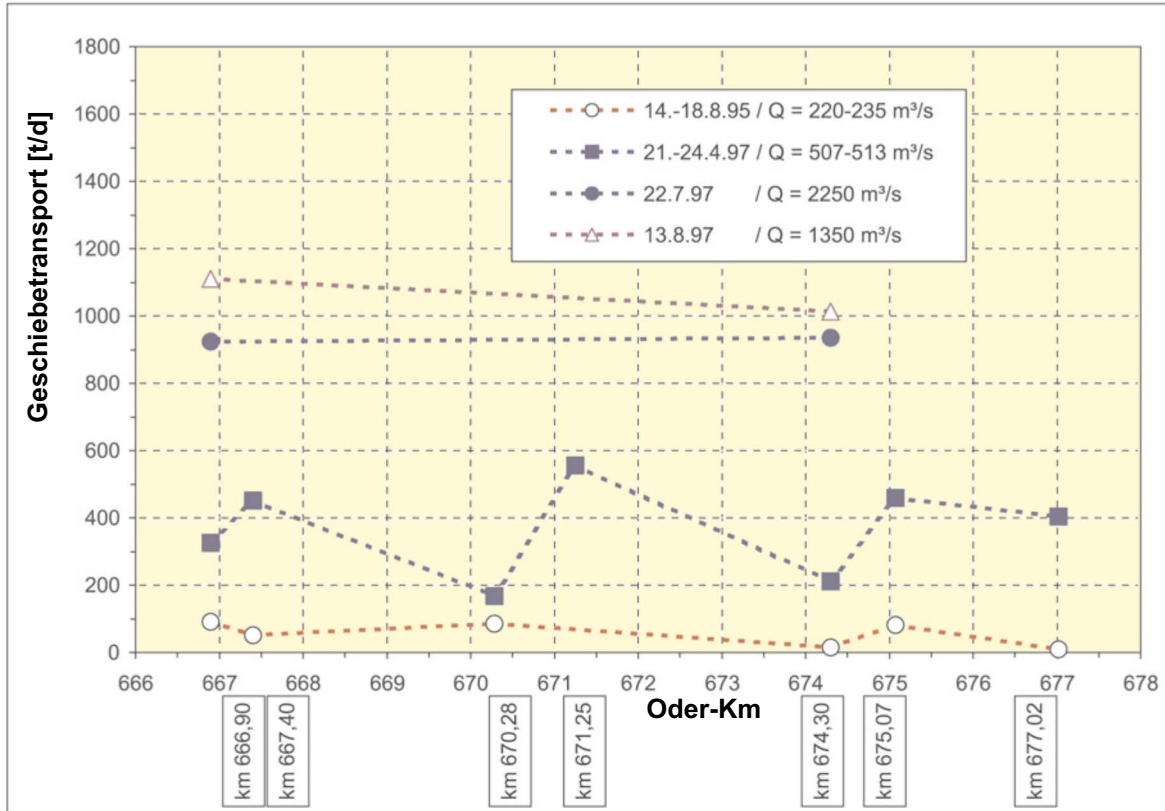
Abb. 8.3 Geschiebetransport im Abschnitt Hohensaaten - Bellinchen
