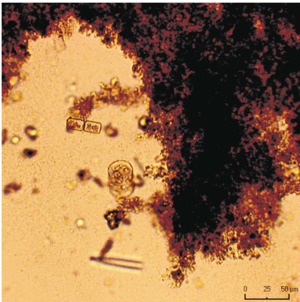
Hochwasserphase (07.08.1997): Starke Aggregation von Wolken feinsten Materials, besonders auffällig in der Zeit des Hochwassers. (125-fache Vergrößerung)
