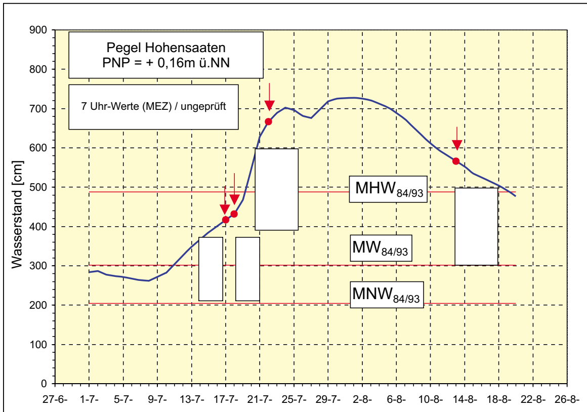
Abb. 8.1b Zeitpunkte der Feststofftransportmessungen bei Hohensaaten
