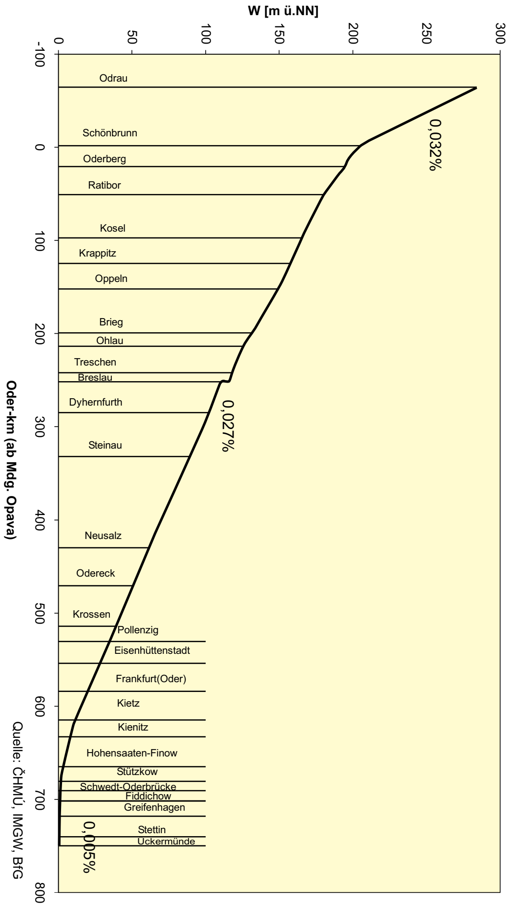
Abb. 2.3 Hydrologischer Längsschnitt der Oder bei MW (mit mittleren Gefälleangaben)
