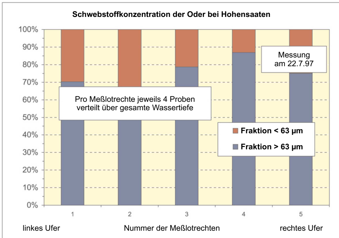
Abb. 8.5b Anteile der Schwebstoffkomponenten bei Hohensaaten am 22.7.1997
