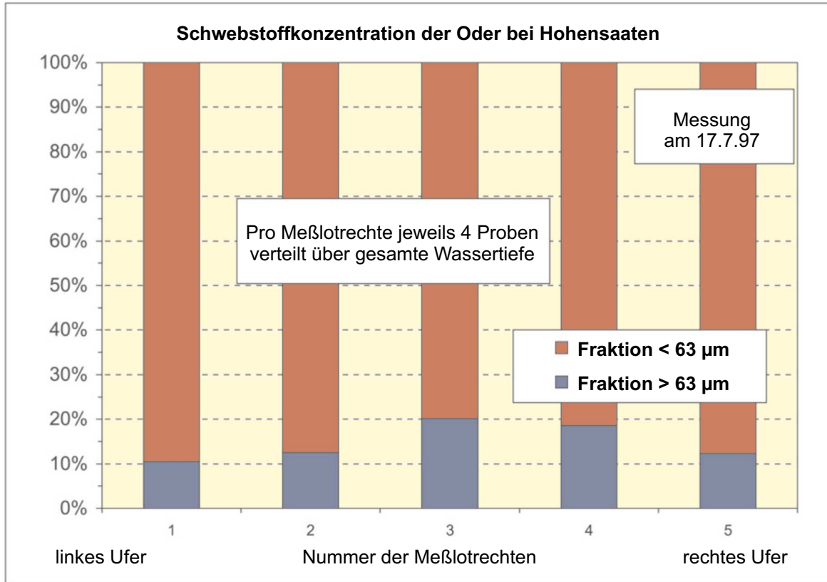
Abb. 8.5a Anteile der Schwebstoffkomponenten bei Hohensaaten am 17.7.1997
