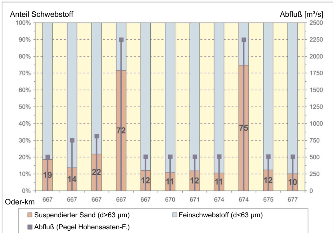
Abb. 8.4 Anteile der Schwebstoffkomponenten bei unterschiedlichen Abflüssen
