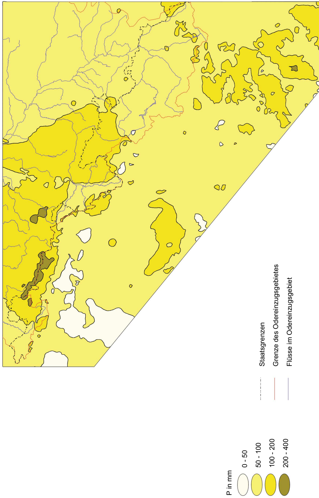
Abb. 3.3 Niederschlagssummen P (17.-21.07.1997)
