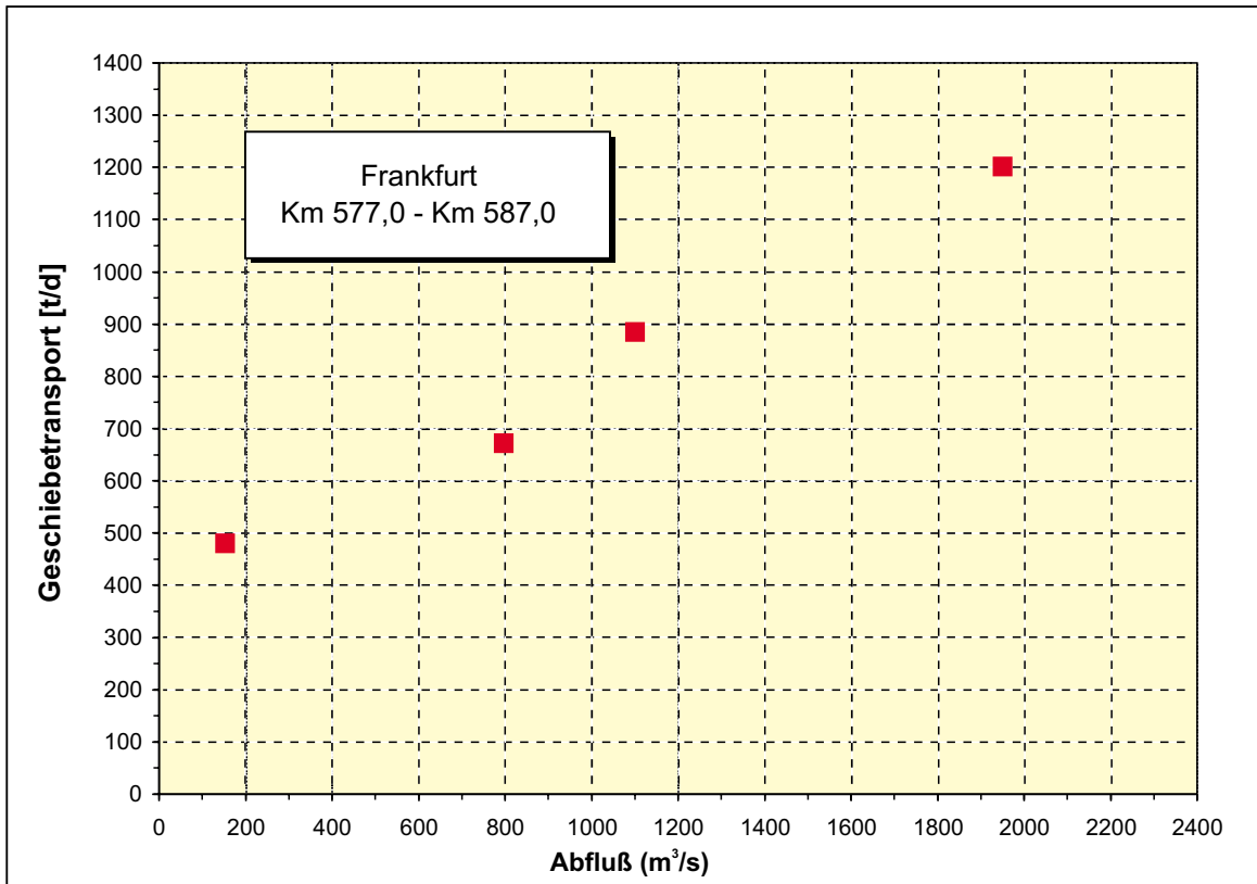
Abb.8.2a Geschiebetransport bei Frankfurt / Oder
